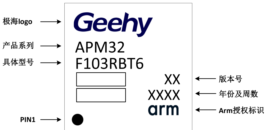
图 25 LQFP64 - 64 引脚，10 x 10mm 封装标识
