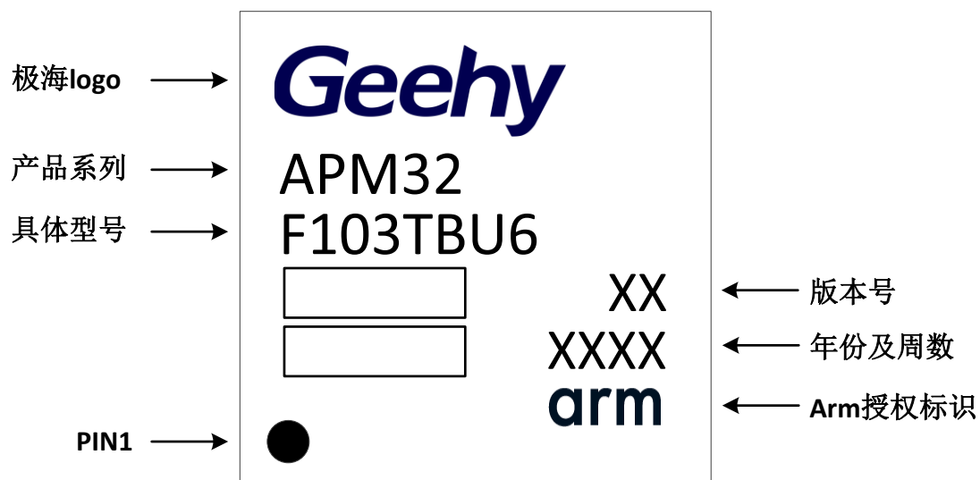
图 31 QFN36 - 36 引脚, 6 x 6 mm 标识图
