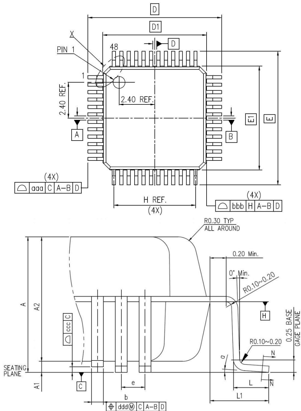
图 26 LQFP48 封装图
