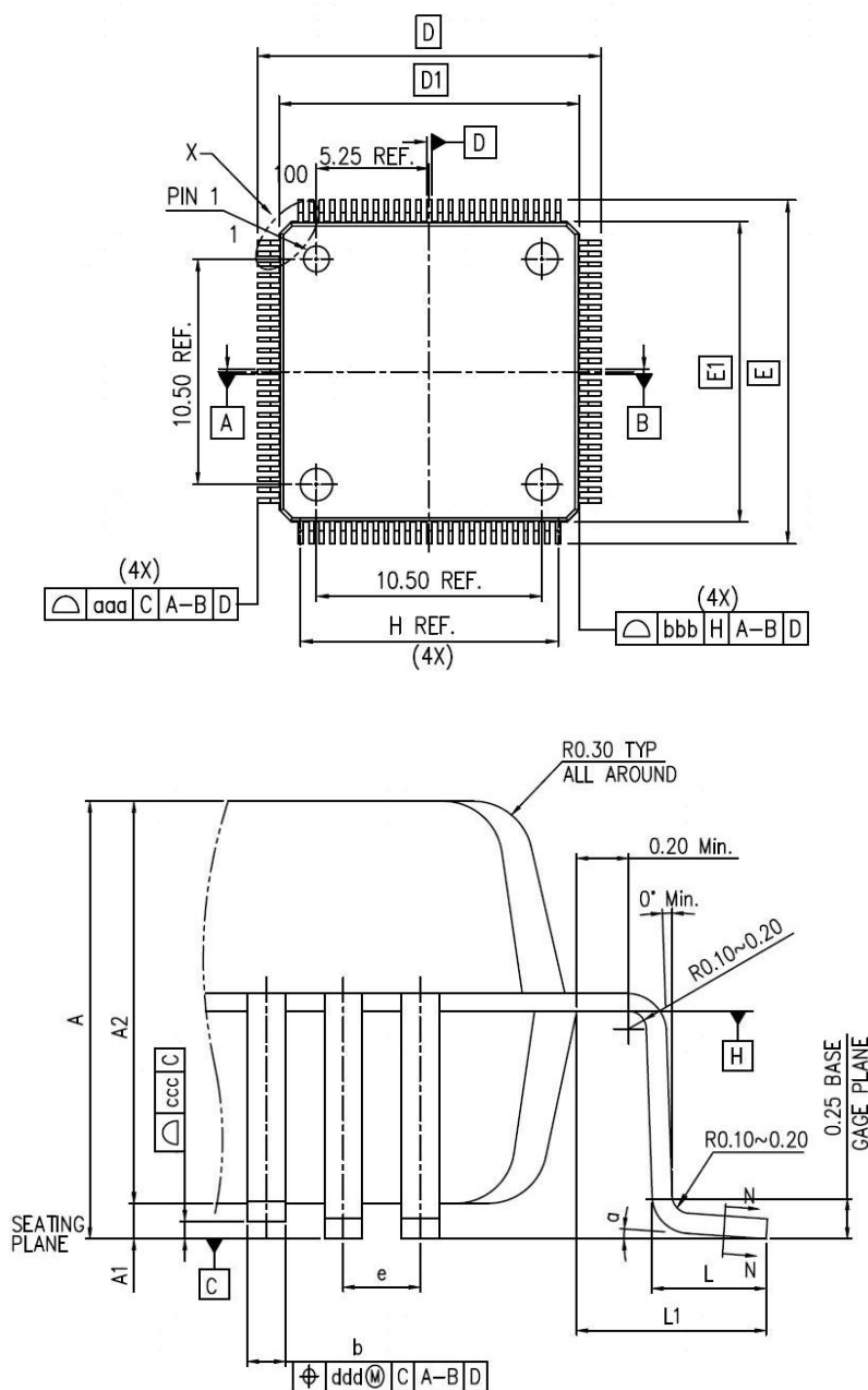
图 20 LQFP100 封装图
